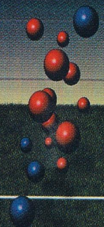
Atoms
